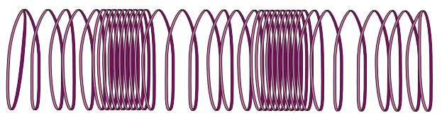
Longitudinal or compression wave
